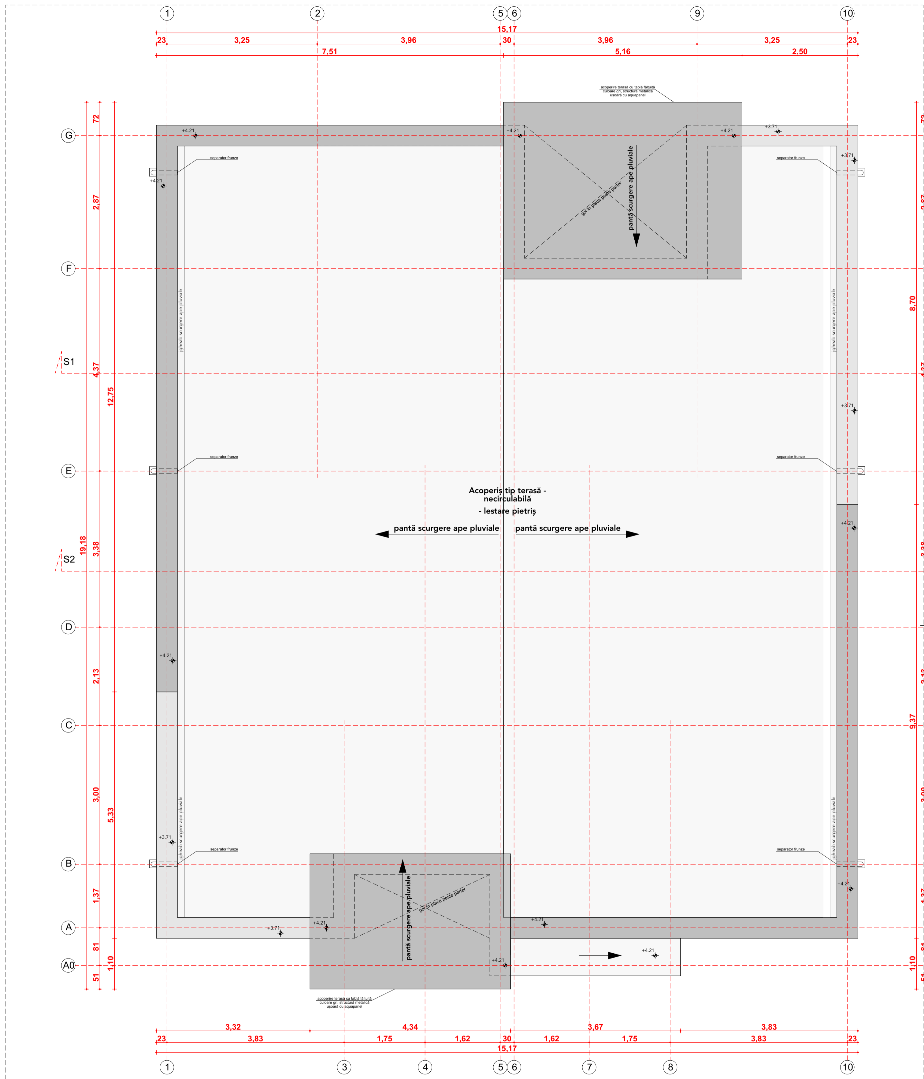
PLAN ÎNVELITOARE
